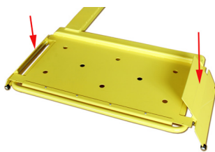
Supporti presa ruote con arresti ruote esterni ed interni
