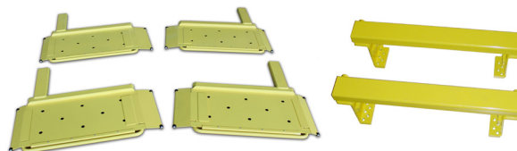
4P – supporti presa ruote con traverse di fissaggio, disponibili come accessorio su tutti i modelli di sollevatori incassati; velocizzano ancora di più il posizionamento del veicolo sul sollevatore ed evitano flessioni della struttura del veicolo stesso
