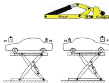
Carico reversibile, la parte più pesante (lato motore) in entrambi i lati
